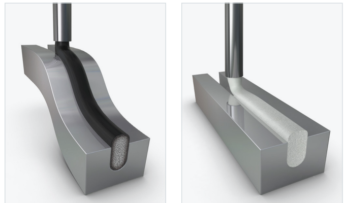
Abdichtung der 2D- oder 3D-Lampengehäusenut mit Polyurethanschaum FERMAPOR K31 oder Silikonschaum FERMASIL
