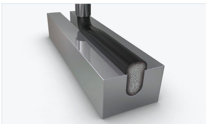
Abdichtung der Leuchtgehäusenut mit Polyurethanschaum FERMAPOR K31
