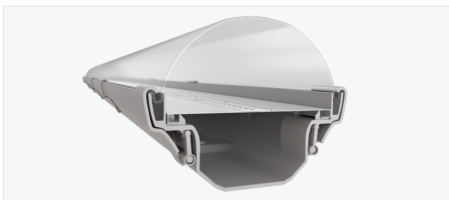
Langfeldleuchte im geschlossenen Zustand, die Dichtung ist komprimiert
