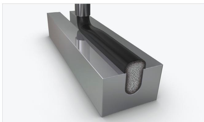
Nutabdichtung der Hinweisleuchte mit Polyurethanschäum FERMAPOR K31
